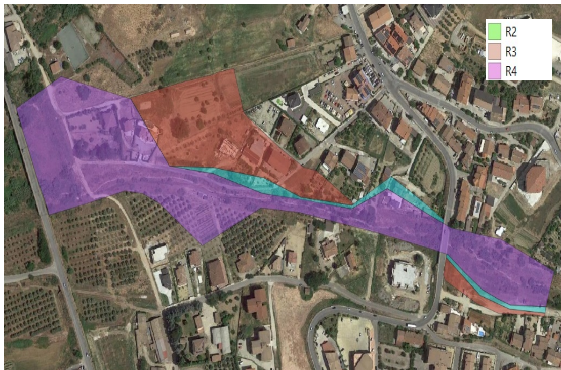
Comune di Luzzi (CS) Torrente Ilice – Stralcio mappa del rischio idraulico - proposta di riperimetrazione
